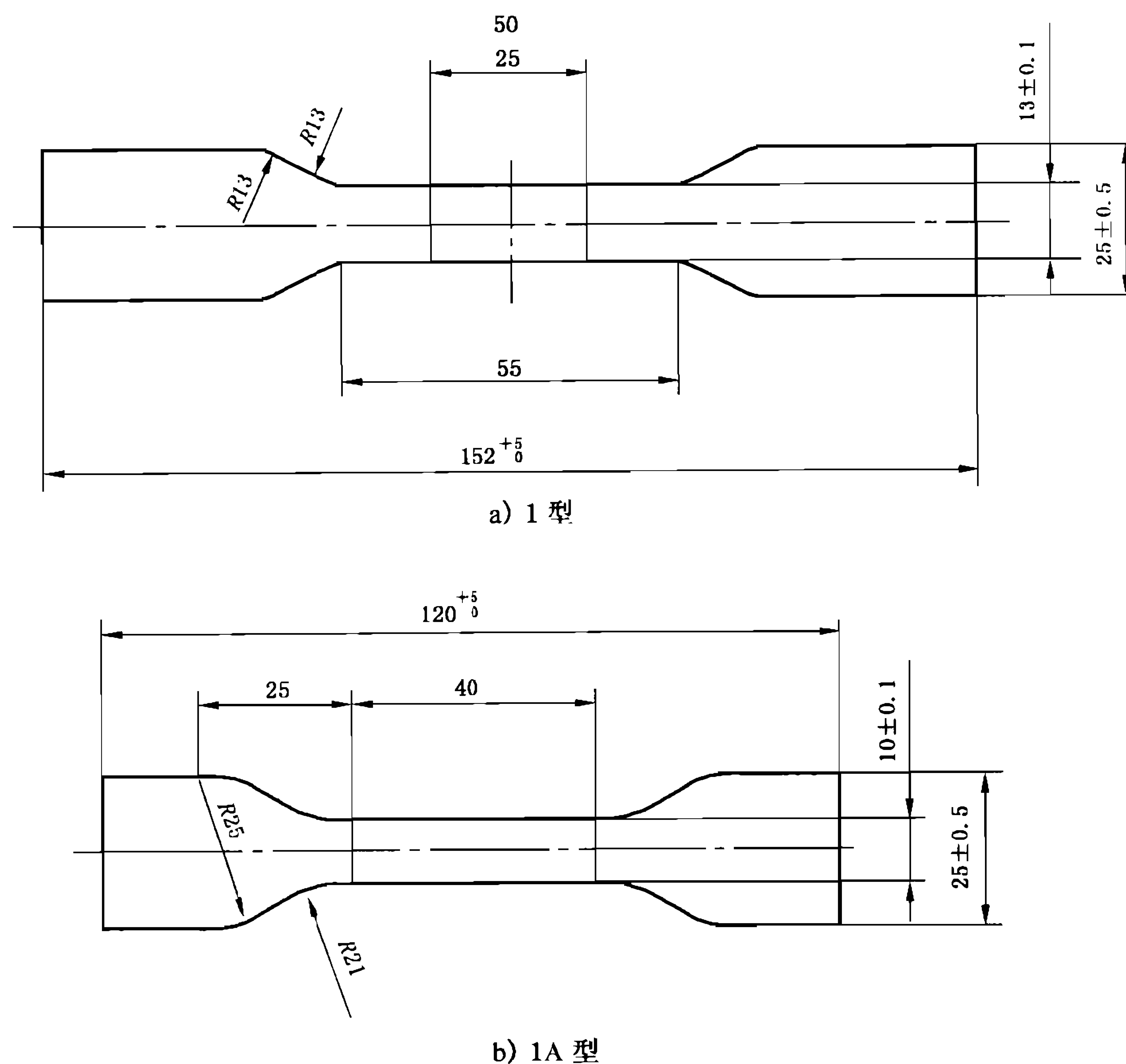
图 1 刀模尺寸示意图
